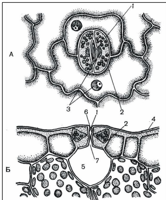
Рисунок 2.1.3.1. Будова продихів
